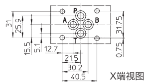
X端视图
