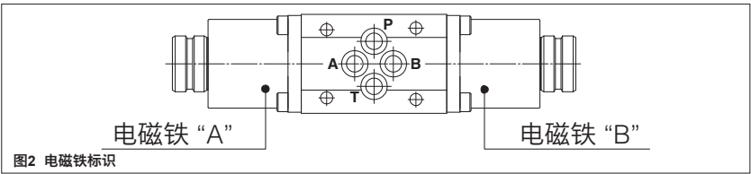
图2 电磁铁标识
